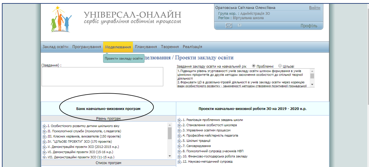
Рис. 7. Рівні програм
